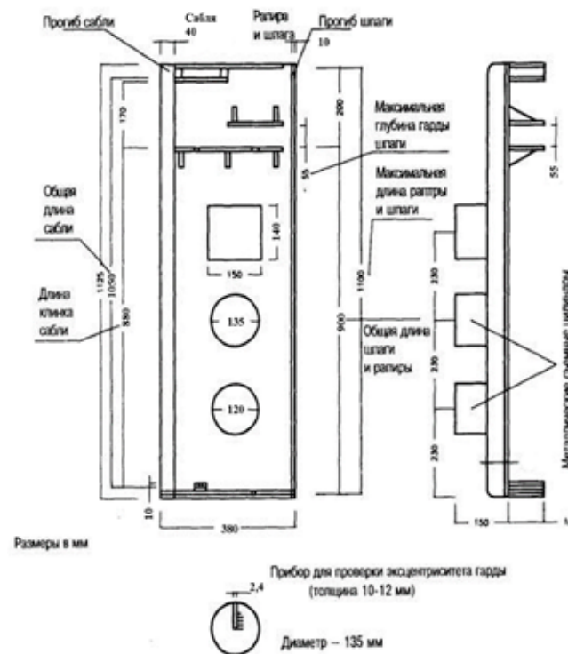
Рисунок 16. Прибор для проверки оружия
