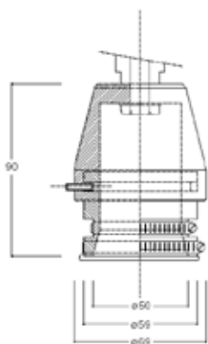
Рисунок А.5. Устройство крепления образцов ткани для испытания одежды на сопротивление к перфорированию
