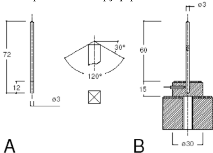
Рисунок А.4. Высокоскоростной динамометр для испытания одежды на сопротивление к перфорированию.
