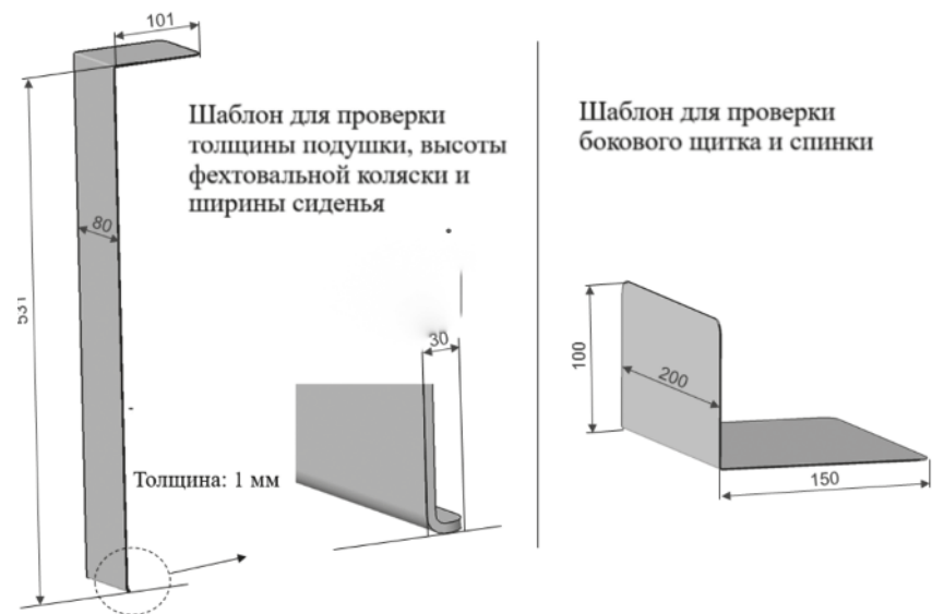
Рисунок 13.2. Шаблоны для тестирования фехтовальной коляски
