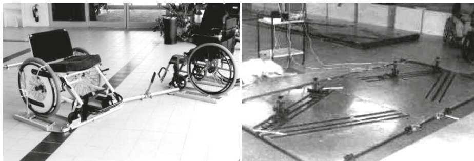
Рисунок 17. Фехтовальные рамы для всех трёх видов оружия
