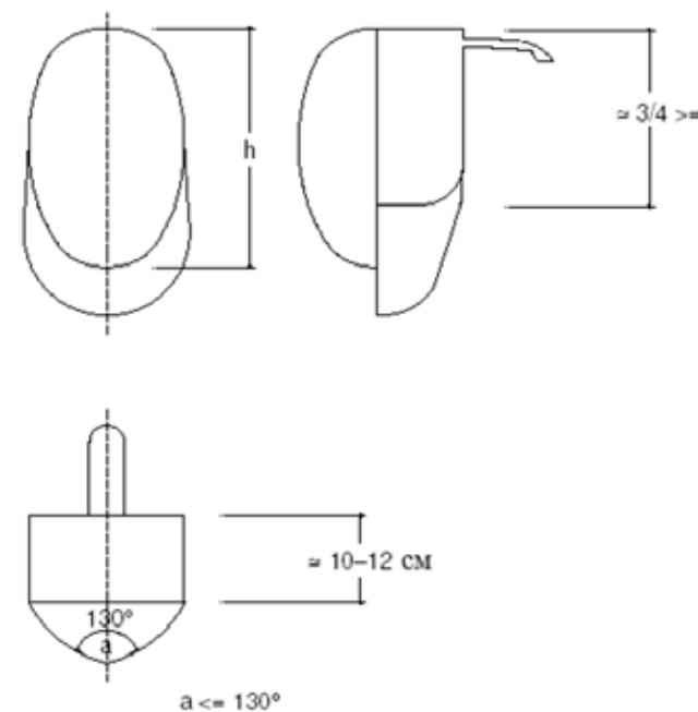
Рисунок А.3. Модель маски
