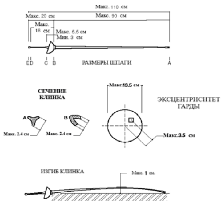
Рисунок 9. Размеры и гибкость шпаги
