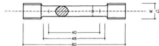
Образец для испытания на растяжение
