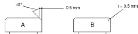
Рисунок 10. Шпага: внешний вид кнопки наконечника
